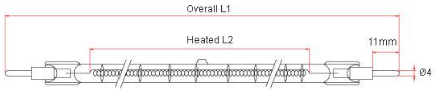
Metal Rod Type
